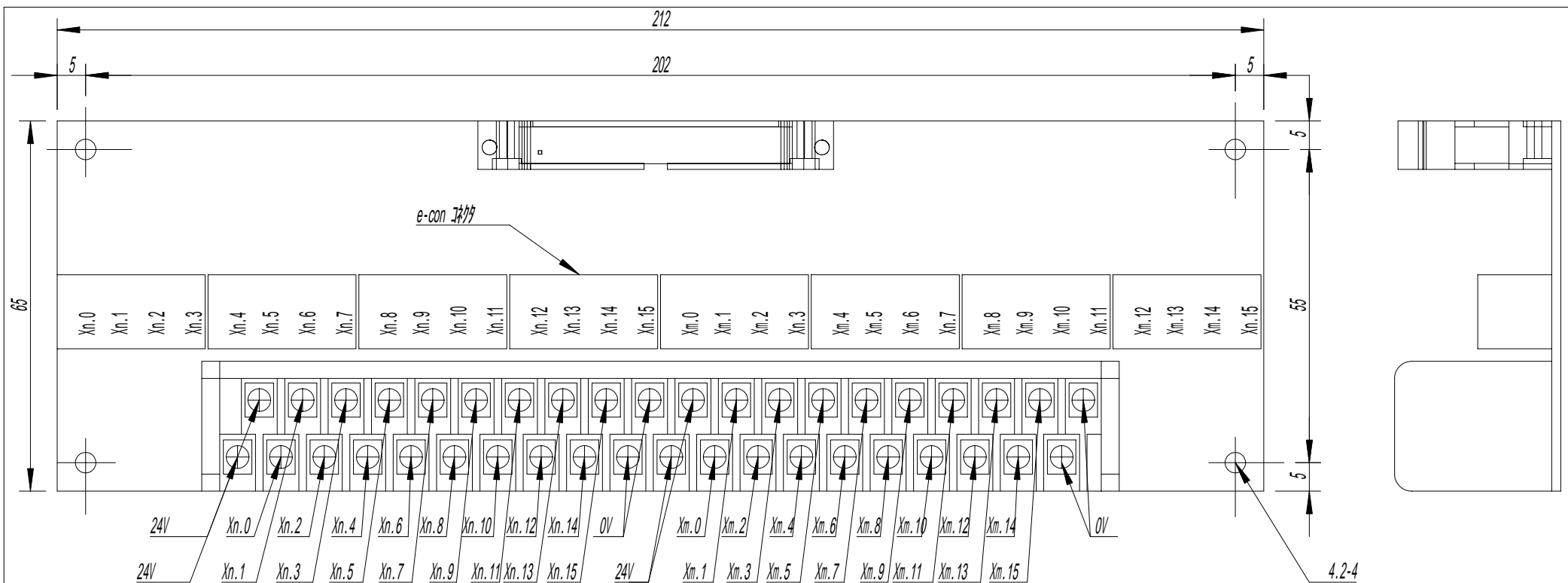
e-Conコネクタピン配置
